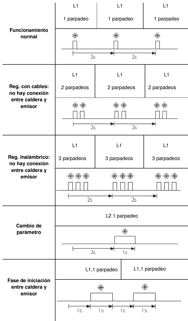
Fig. 27: LEDs del estado de sincronización del receptor
