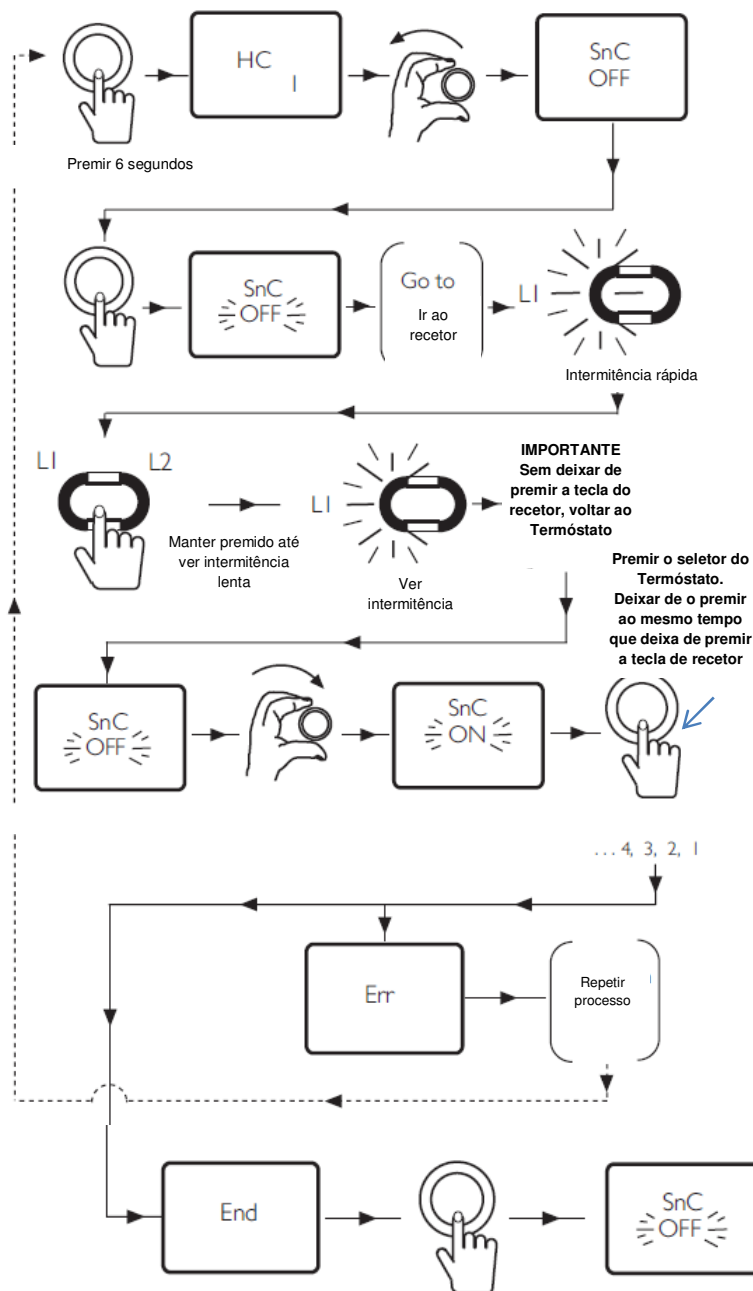
Fig. 17: Diagrama do processo de sincronização manual
